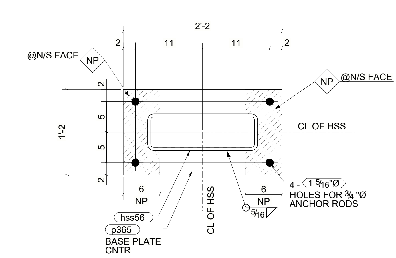
B-B
