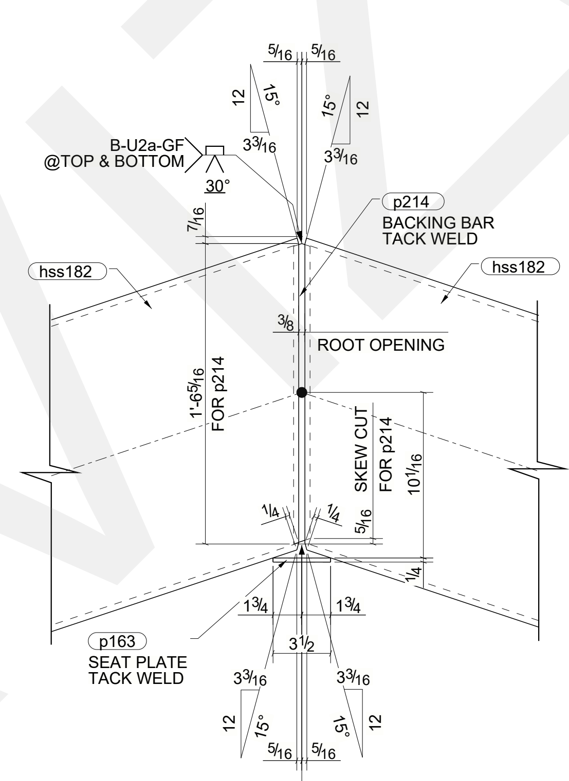
DETAIL-B
